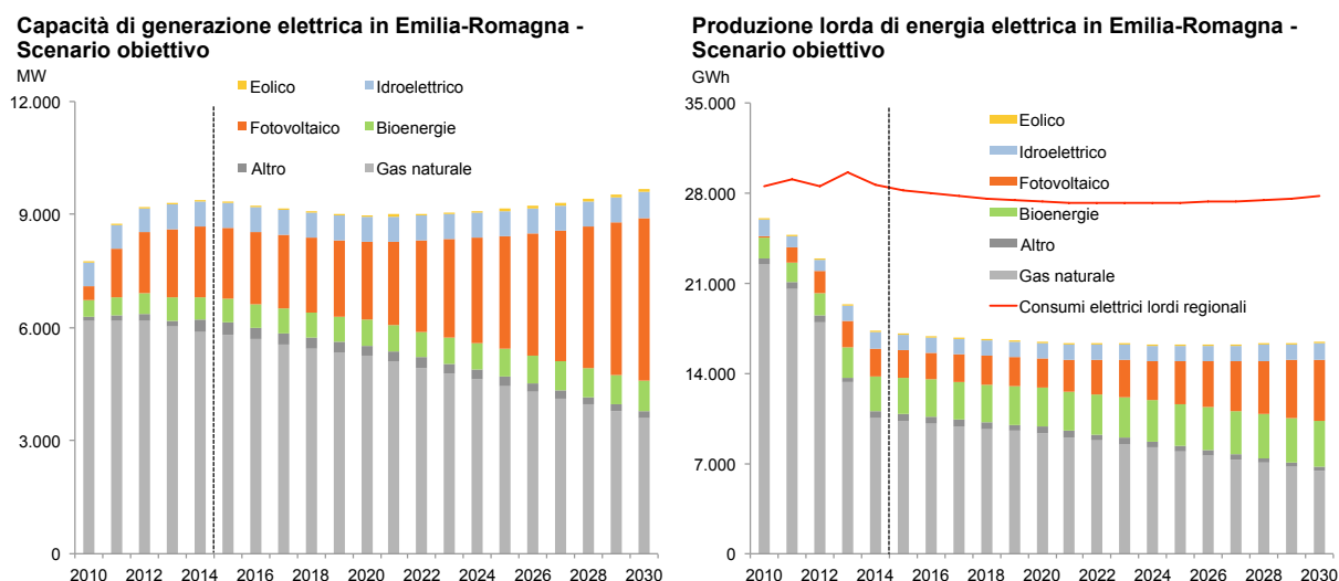
Figura 23 - Scenario obiettivo del parco di generazione elettrica in Emilia-Romagna al 2030
