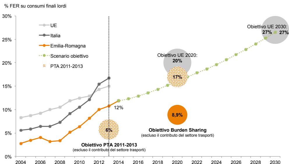
Figura 35 - Raggiungimento degli obiettivi di copertura dei consumi finali lordi con fonti rinnovabili nello scenario energetico obiettivo per l'Emilia-Romagna al 2030
