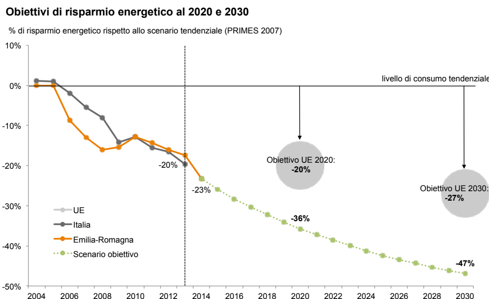
Figura 34 - Raggiungimento degli obiettivi di risparmio energetico nello scenario energetico obiettivo per l'Emilia-Romagna al 2030
