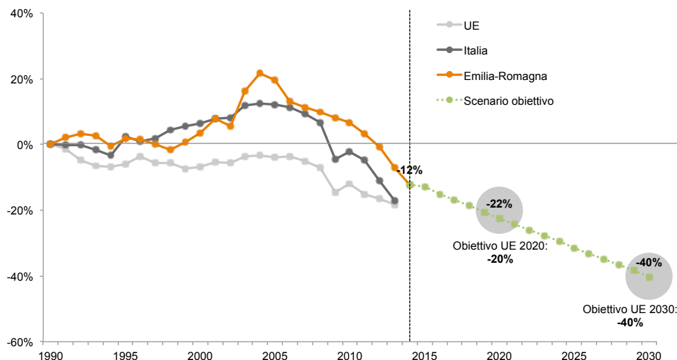
Figura 33 - Raggiungimento degli obiettivi di riduzione delle emissioni serra nello scenario energetico obiettivo per l'Emilia-Romagna al 2030
