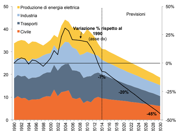
Figura 30 - Scenario obiettivo delle emissioni di CO 2 da combustione in Emilia-Romagna al 2030 28
