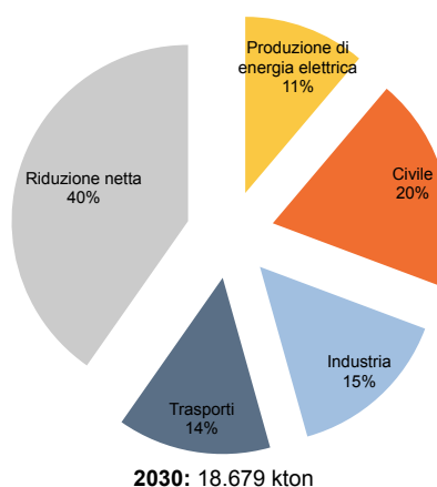
Figura 30 - Scenario obiettivo delle emissioni di CO 2 da combustione in Emilia-Romagna al 2030 28
