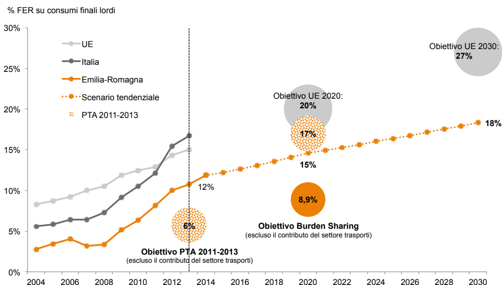
Figura 21 - Raggiungimento degli obiettivi di copertura dei consumi finali lordi con fonti rinnovabili nello scenario energetico tendenziale per l'Emilia-Romagna al 2030
