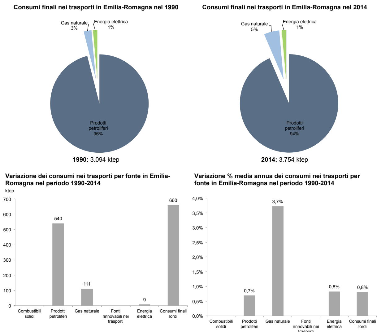
Figura 13 - Consumi nei trasporti in Emilia-Romagna nel periodo 1990-2014
