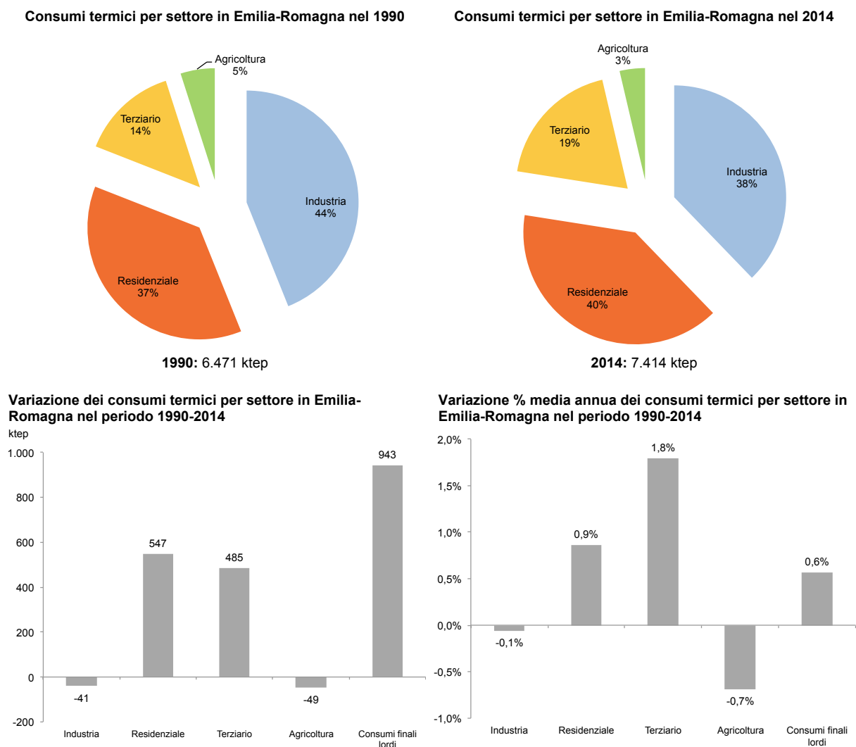
Figura 11 - Consumi per riscaldamento e raffrescamento in Emilia-Romagna nel periodo 1990-2014
