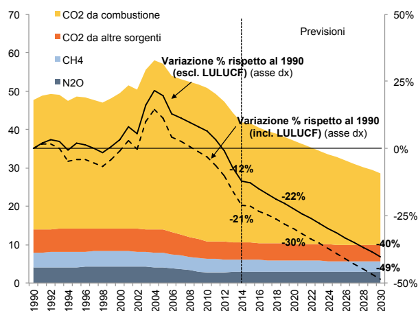
Figura 29 - Scenario obiettivo delle emissioni di gas serra in Emilia-Romagna al 2030 27
