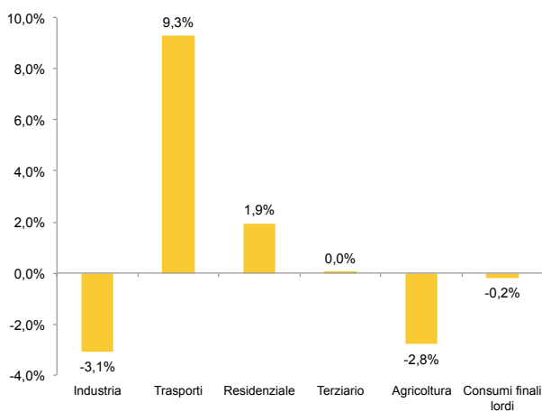
Variazione % media annua dei consumi elettrici per settore in Emilia-Romagna nel periodo 2014-2030 - Sc. obiettivo
