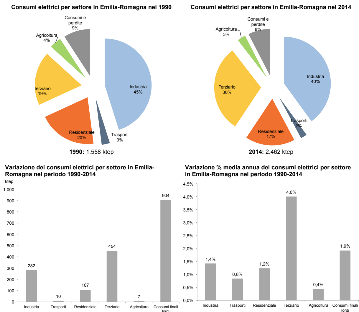
Figura 9 - Consumi elettrici in Emilia-Romagna nel periodo 1990-2014
