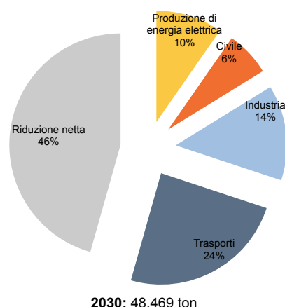
Figura 32 - Scenario obiettivo delle emissioni di ossidi di azoto in Emilia-Romagna al 2030 30
