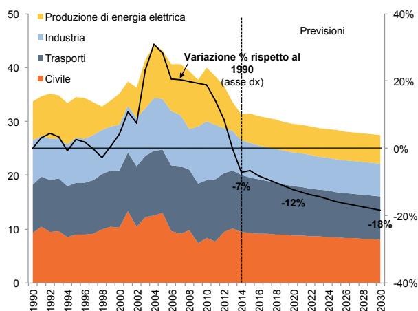
Figura 16 - Scenario tendenziale delle emissioni di CO 2 da combustione in Emilia-Romagna al 2030 14
