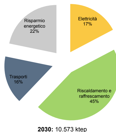
Figura 25 - Scenario obiettivo dei consumi finali lordi per settore in Emilia-Romagna al 2030 22
